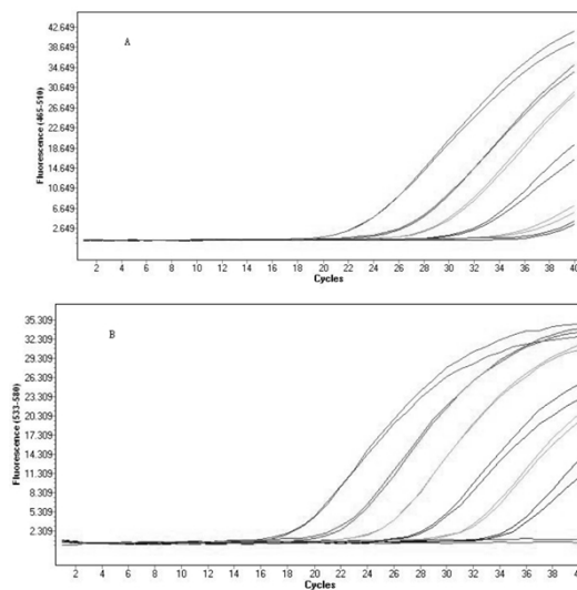
图 1 双重荧光 RT-PCR 方法敏感性检测 A. AKAV-FAM; B.SBV-VIC
